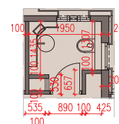
PART PLANS SHOWING LATEST LAYOUT 現狀間隔部分平面圖
