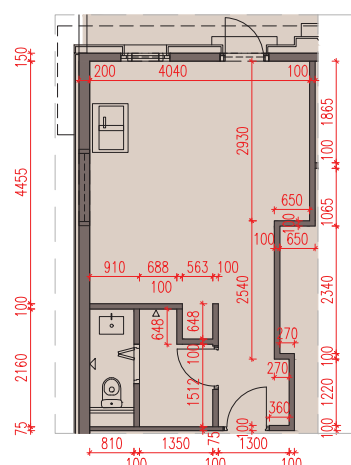
PART PLANS SHOWING LATEST LAYOUT 現狀間隔部分平面圖
