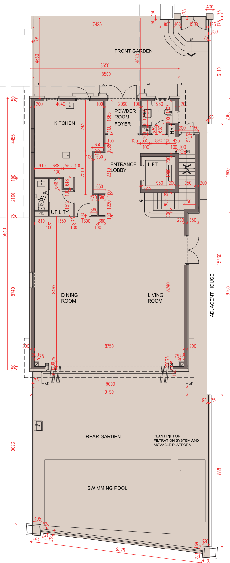
PART PLANS SHOWING LATEST LAYOUT 現狀間隔部分平面圖
