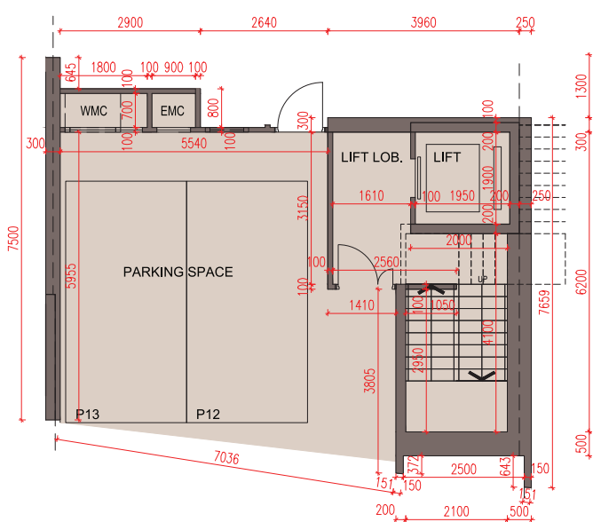
LOWER GROUND FLOOR PLAN 地下低層平面圖
