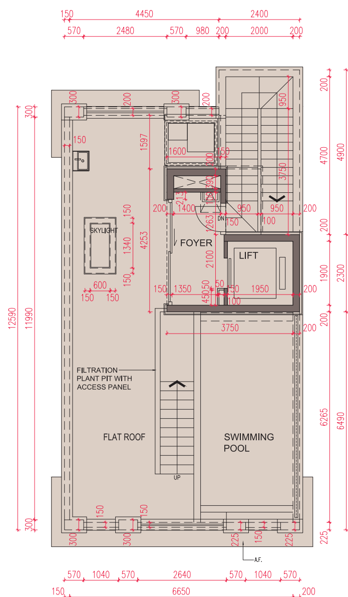
ROOF FLOOR PLAN 天台平面圖
