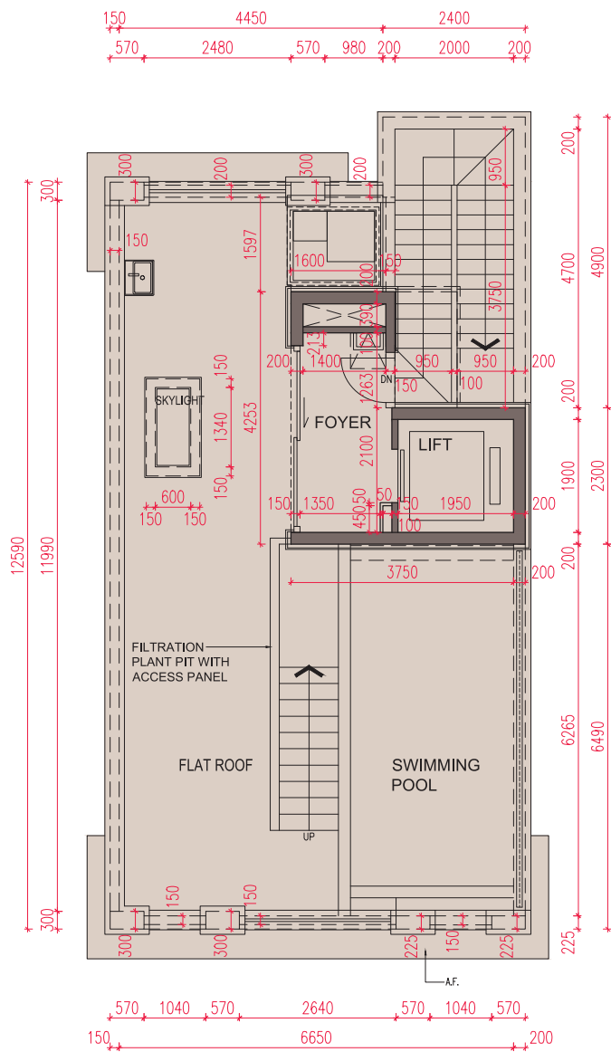
ROOF FLOOR PLAN 天台平面圖
