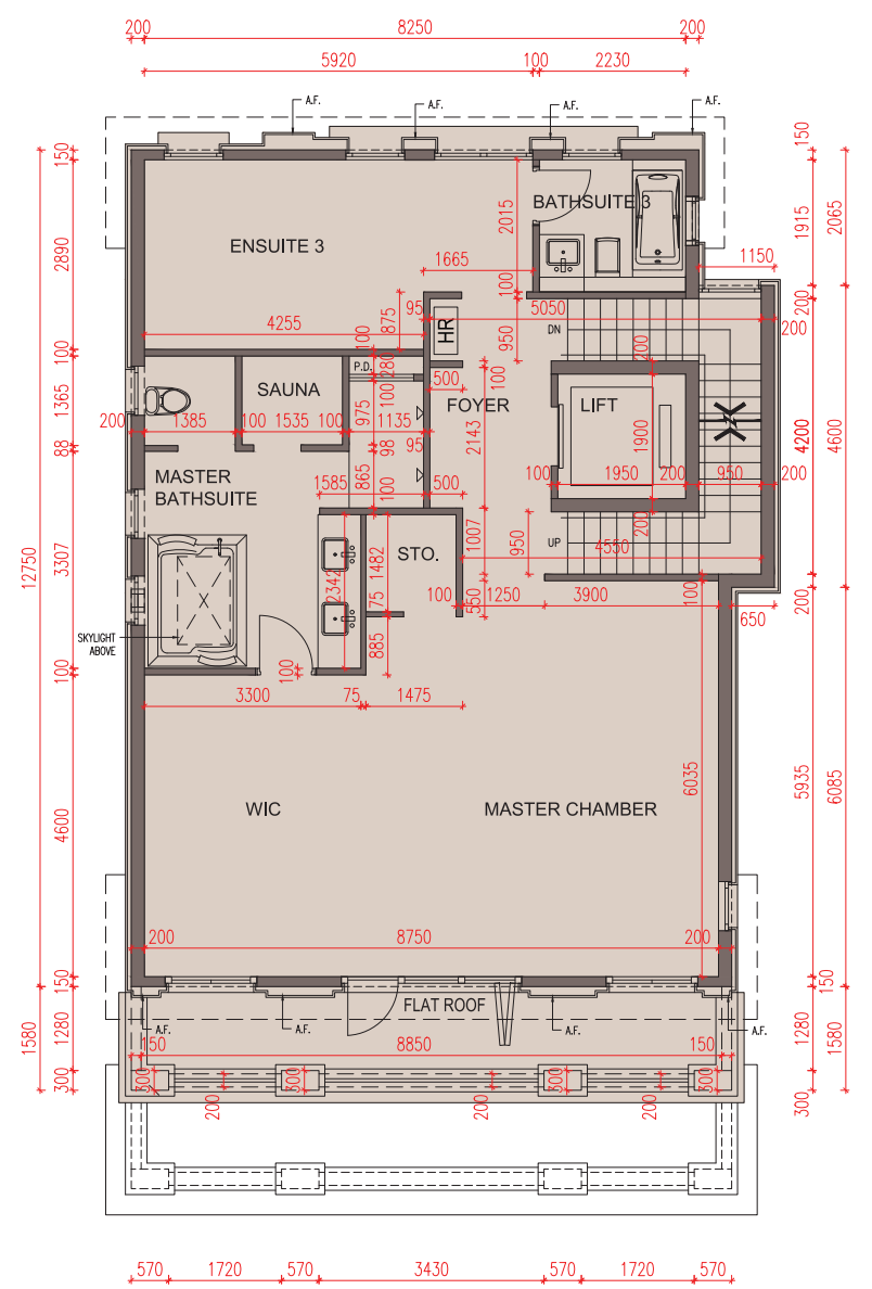
SECOND FLOOR PLAN 二樓平面圖
